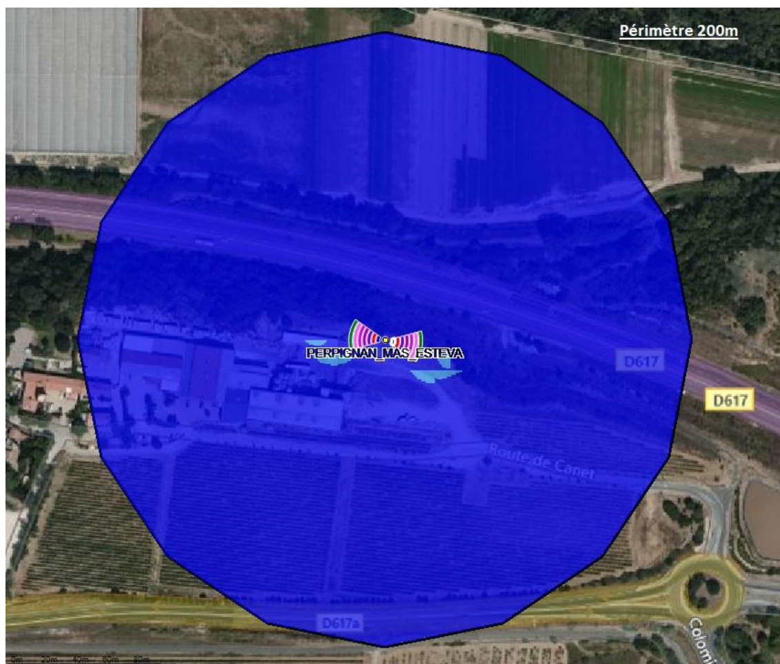
Fond de carte (photo aérienne), source : bing. Logiciel de simulation Cellergy, éditeur Orange Labs
